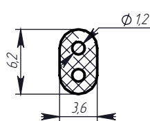
Профиль № 630
