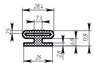
Профиль № 101
