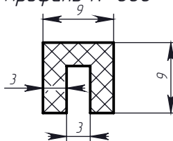
Профиль № 860
