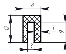
Профиль № 570
