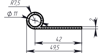
Профиль № 416
