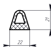
Профиль № 717
