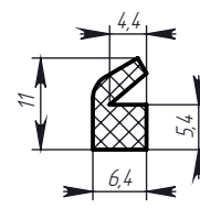
Профиль № 664
