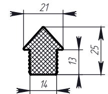
Профиль № 507
