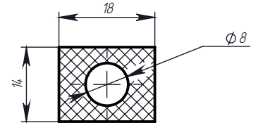
Профиль № 485
