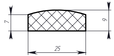
Профиль № 139
