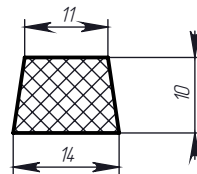
Профиль № 525
