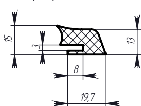
Профиль № 105
