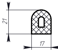
Профиль № 563
