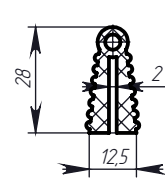
Профиль № 718
