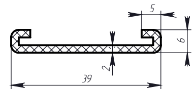
Профиль № 847
