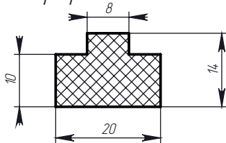
Профиль № 883
