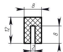
Профиль № 529
