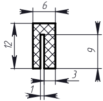
Профиль № 579
