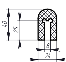
Профиль № 709
