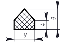
Профиль № 475
