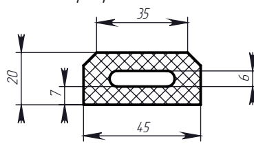
Профиль № 108
