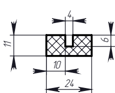
Профиль № 667
