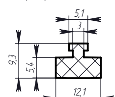
Профиль № 735
