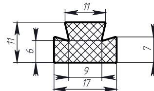
Профиль № 946
