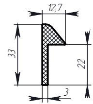
Профиль № 433
