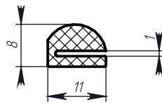
Профиль № 566
