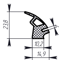
Профиль № 688
