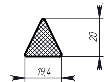
Профиль № 521
